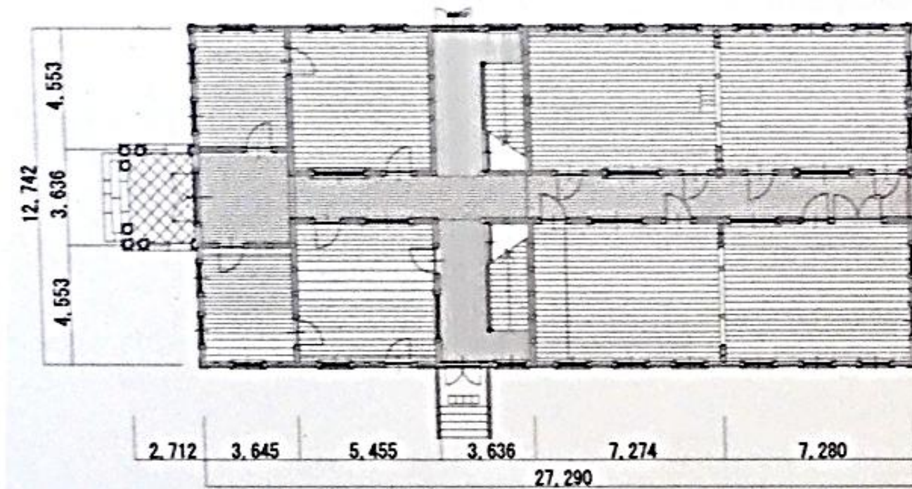
1 階平面図
