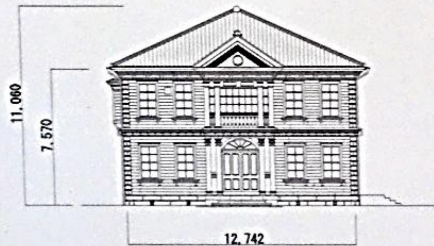
西立面図
