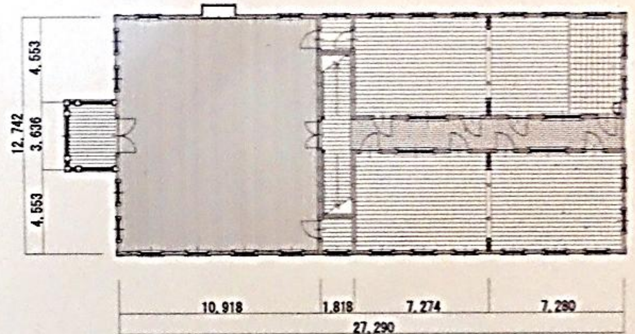
2 階平面図
